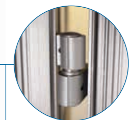
PAUMELLES THERMOLAQUÉES COULEUR PORTE : RÉGLAGE SUR 3 AXES : HAUTEUR, LARGEUR ET COMPRESSION
